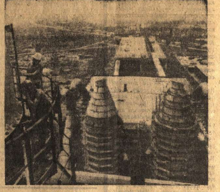
ВЕНТЕРСКАЯ НАРОДНАЯ РЕСПУБЛИКА. В Хещебае (область Боршол) строятся самый большой цементный завод страны. По достижении проектной мощности он будет давать в год 1,6 миллиона тонн цемента. Над строительством завода шефствуют комсомольцы области. НА СНИМКЕ: вид на один из участков строительства завода. Фото МТИ — АИП.
