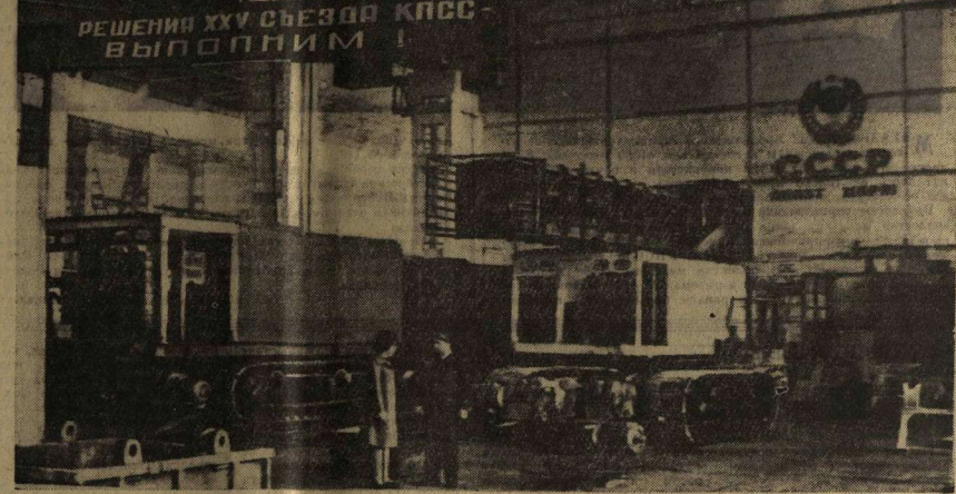
ВЫПУСКАЕМЫЙ заводом станок с диаметром бурения 230 миллиметров. Упомянутый в решении XXV съезда КПСС. В текущем пятилетии коллектив обогатительного цеха № 4 приступит к созданию новой машины с диаметром бурения 400 миллиметров. Конструкторы уже приступили к проектированию работ по созданию новой машины. Фото В. Майорова.
