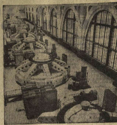
ВОЛХОВ (Ленинградская область). 19 декабря исполняется 50 лет со дня пуска первого Ленинского плана ГОЭЛРО — Волховской ГЭС. Ветер отечественной энергетики переживает сейчас второе рождение. После реконструкции мощность станции значительно увеличится.
