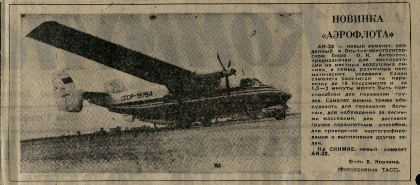
АН-28 — новый самолет, созданный в Опытном конструкторском бюро О. К. Антонова. Предназначен для эксплуатации в условиях самых различных климатических условий. Салон самолета рассчитан на перевозку до 18 пассажиров и за 15-20 минут может быть приспособлен для перевозки грузов. Самолет можно также оборудовать для перевозки больных. Для наблюдений за лесными пожарами самолет может быть оборудован парашютным способом, для проведения картографирования и выполнения других задач.
