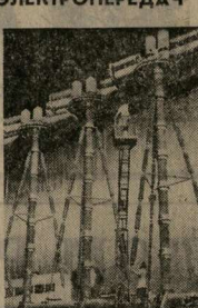
Свердловск. В сверхмасштабной лаборатории научно-исследовательского института промышленного объединения «Уралэлектротехника» закончены испытания опытного образца циркулярной в нашей стране воздушного выключателя высокого напряжения. Он предназначен для магистральных линий электропередачи напряжением 1,1 миллиона вольт. Выключатель — 150 тысяч вольт. Выключатель — 150 тысяч вольт. Выключатель — 150 тысяч вольт.
