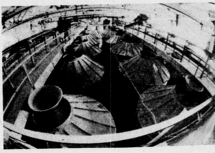
Реактор для предпосевной обработки семян зерновых озонот создан в Новгородском НИИ сельского хозяйства. Эта операция на 9 процентов повышает всхожесть и на 20 процентов увеличивает энергию посевного материала, одновременно происходит обеззараживание семян.
