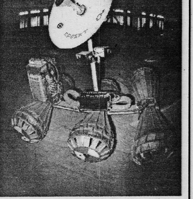
Первый опытный образец ходовой части марсохода разработали специалисты Санкт-петербургского ВНИИ «Трансман». После всесторонних испытаний он будет представлен для демонстрации ученым в США, занимающимся космическими проблемами.
