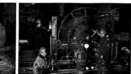
■ Сборка коллибинговой установки «Уран-20» для ремонта нефтяных скважин.
