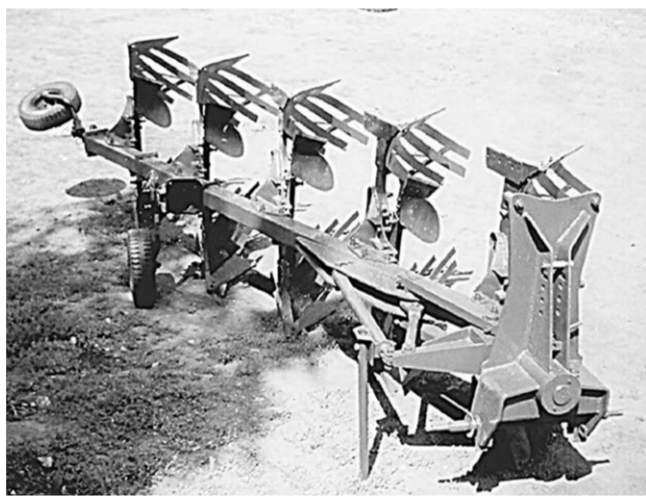
Навесной оборотный плуг ПОН 4-45(+1).
