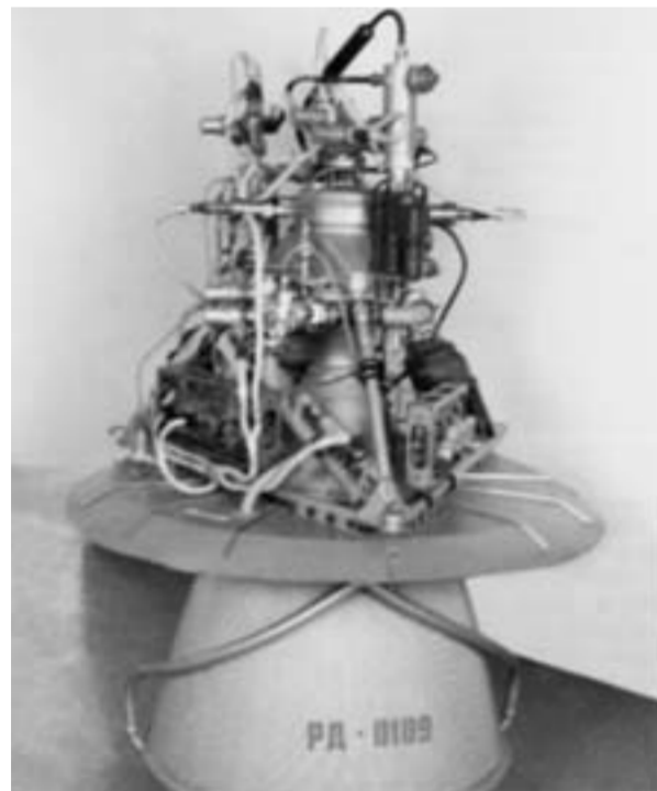
Этот двигатель ВМЗ вывел в космос «Восток» Юрия Гагарина.
