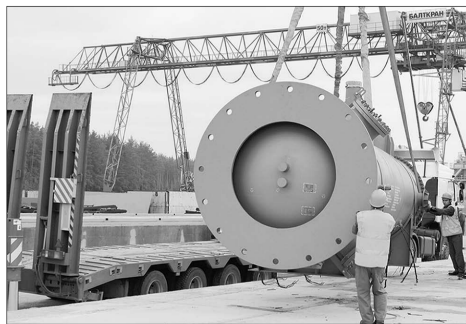
Идёт разгрузка подогревателей сетевой воды.
