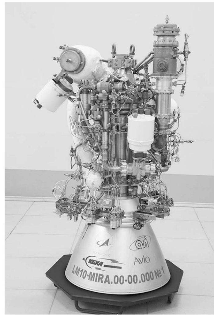
Двигатель LM10-MIRA.
