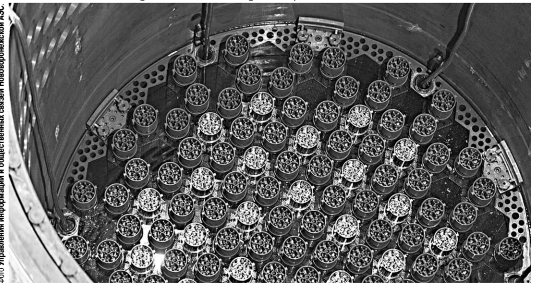
Активная зона реактора ВВЭР-1200 с загруженным топливом.
