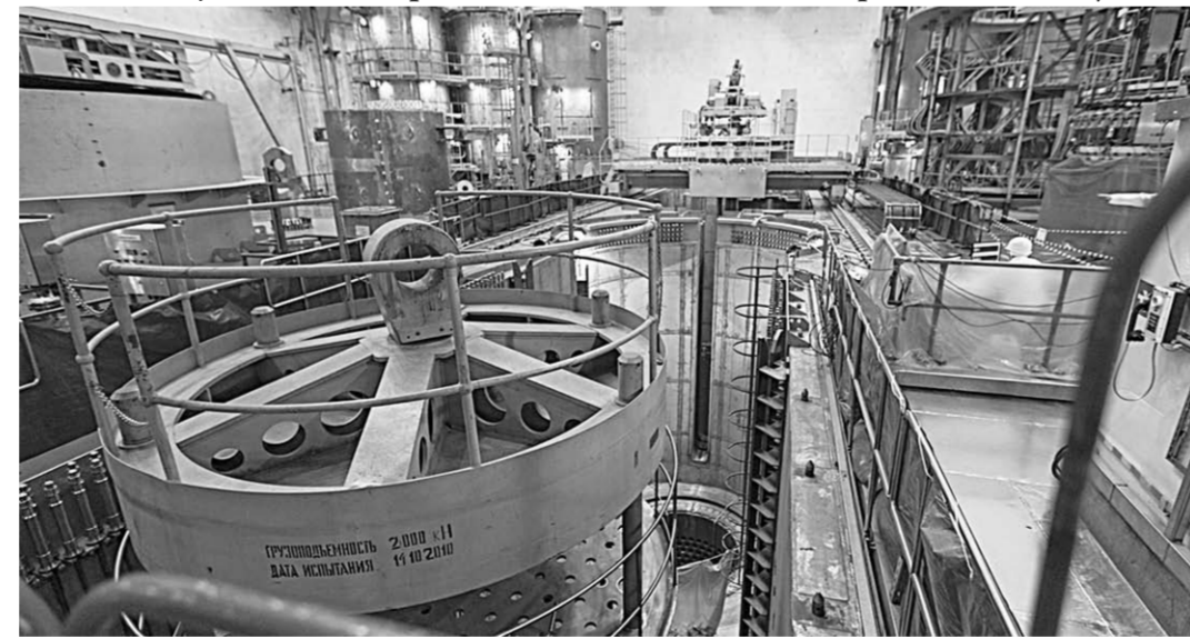
Общий вид центрального зала реакторного отделения.
