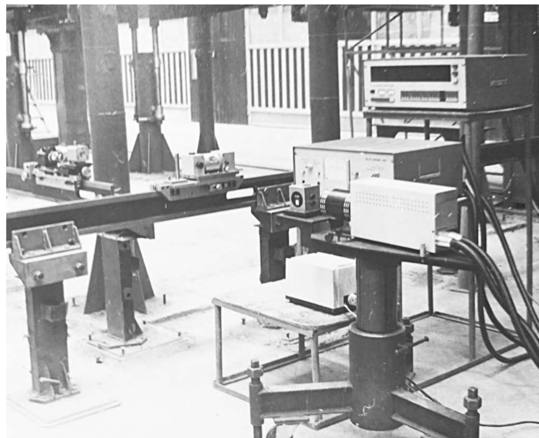
Монтаж стاپеля крыла Ил-96 с помощью лазерной системы ГАПСИ-1.
