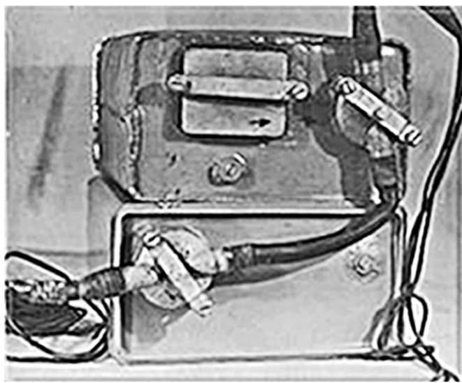
Прибор Ф-40 для управления радиофугасами стратегического назначения.
