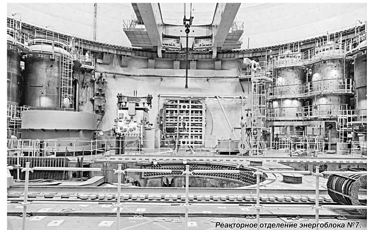
Реакторное отделение энергоблока №7.
