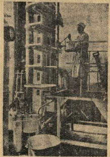
Новосибирск. Шоколадная фабрика имени Героев Сталинграда оснащается новейшей техникой. Недавно здесь смонтирован и пущен мощный пресс, на котором изготавливается из бобов какао-масло. Эта машина и двадцать пять раз производительнее применявшейся ранее. Коллектив фабрики за четыре месяца выпустил более чем на сотню миллионов рублей продукции сверх плана. На снимке: прессыоник И. В. Свинокроз за работой на новом прессе. За смену он вырабатывает до 800 килограммов какао-масла. Фото В. Лещинского (ТАСС).
