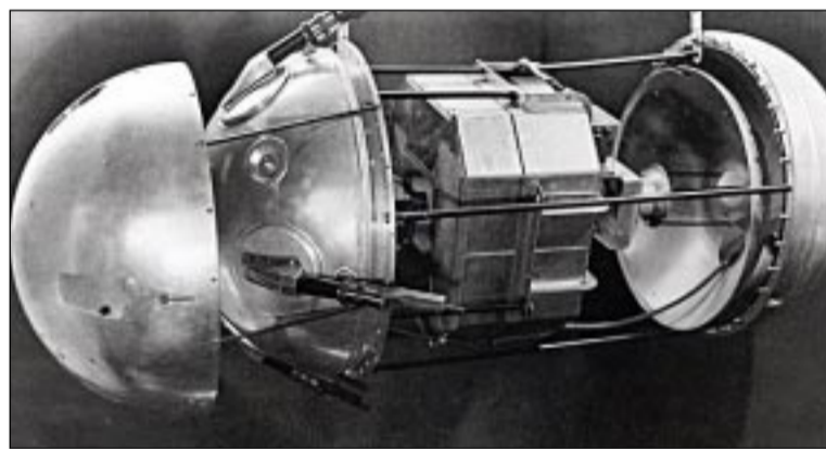
Спутник ПС-1 был устроен довольно просто: внутри у него почти ничего не было, кроме радиостанции, посылающей сигналы на Землю, и источников питания. Фото: NASA
